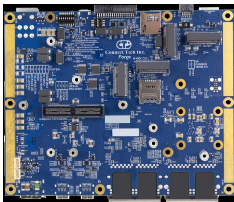
AGX201Forge キャリアボード (AGX Orin 32GB)
